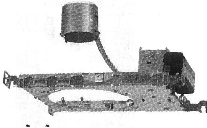
LIGHTOLIER 1002F1 COMPACT FLUORESCENT
